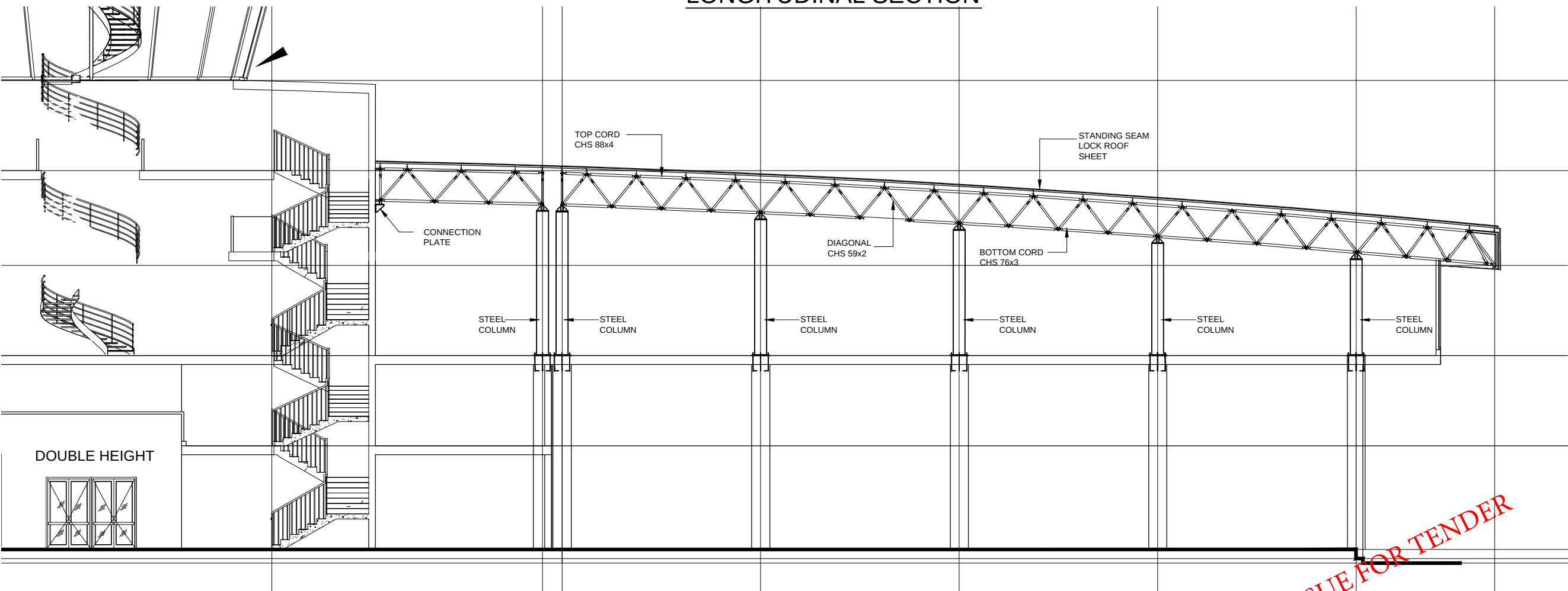
LONGITUDINAL SECTION
