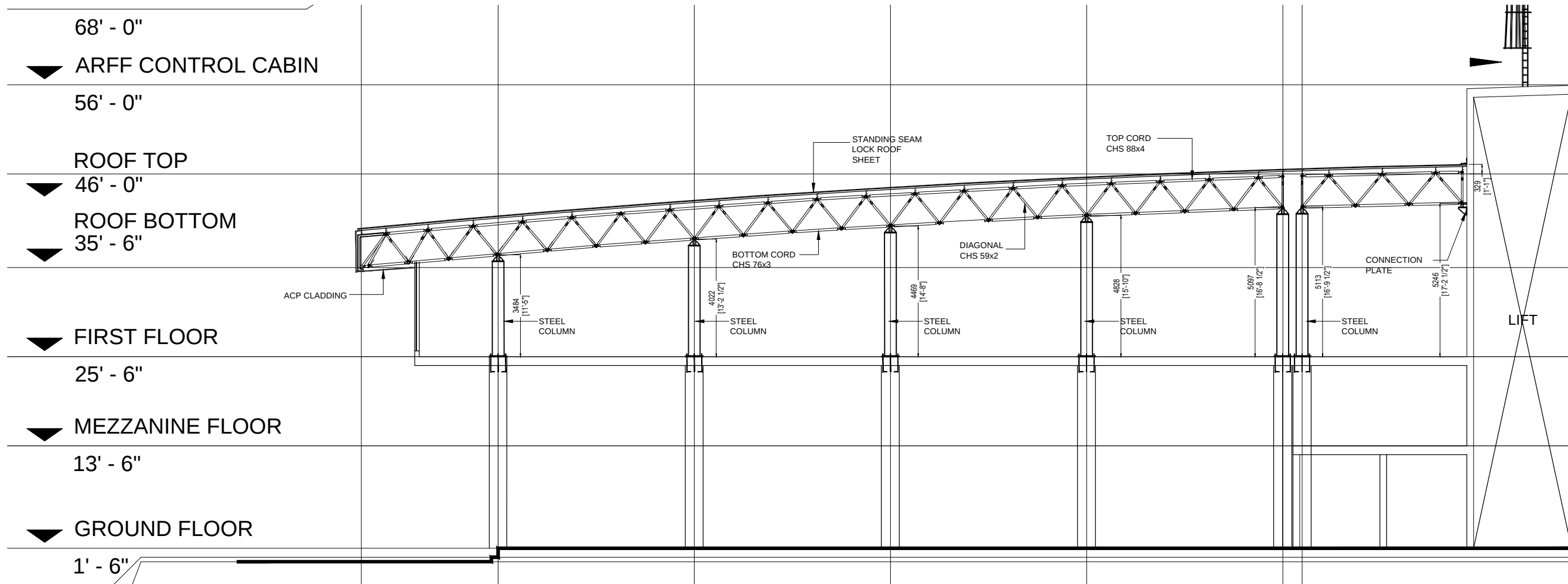
LONGITUDINAL SECTION
