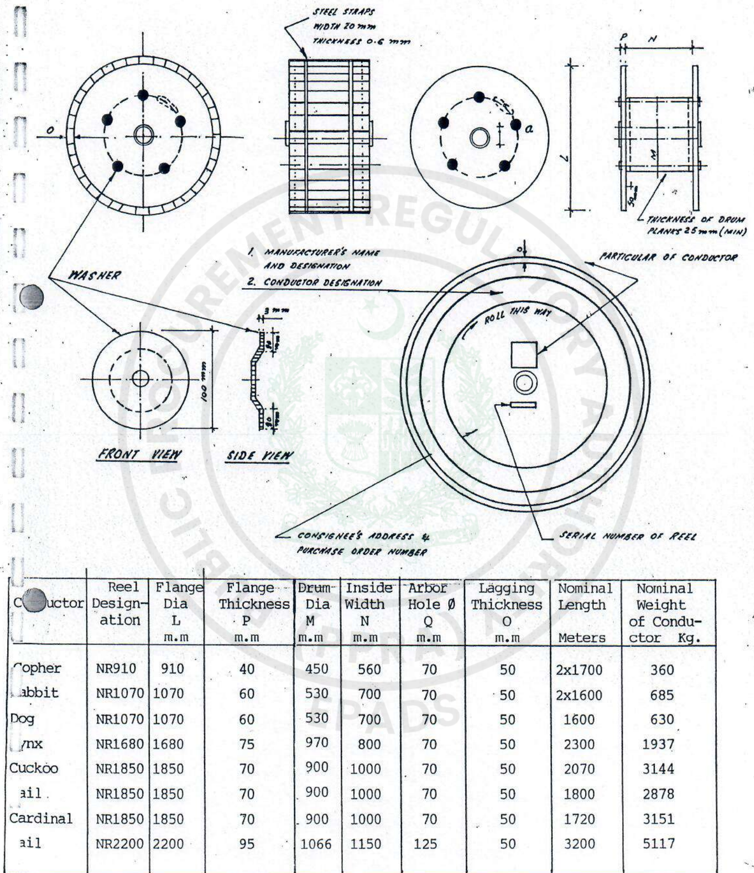
FIG. 1 REEL DIMENSIONS
