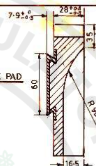
SEC: A-A
