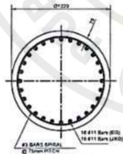
SECTION D-D
