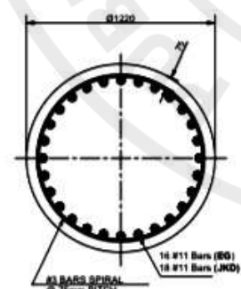
SECTION D-D
