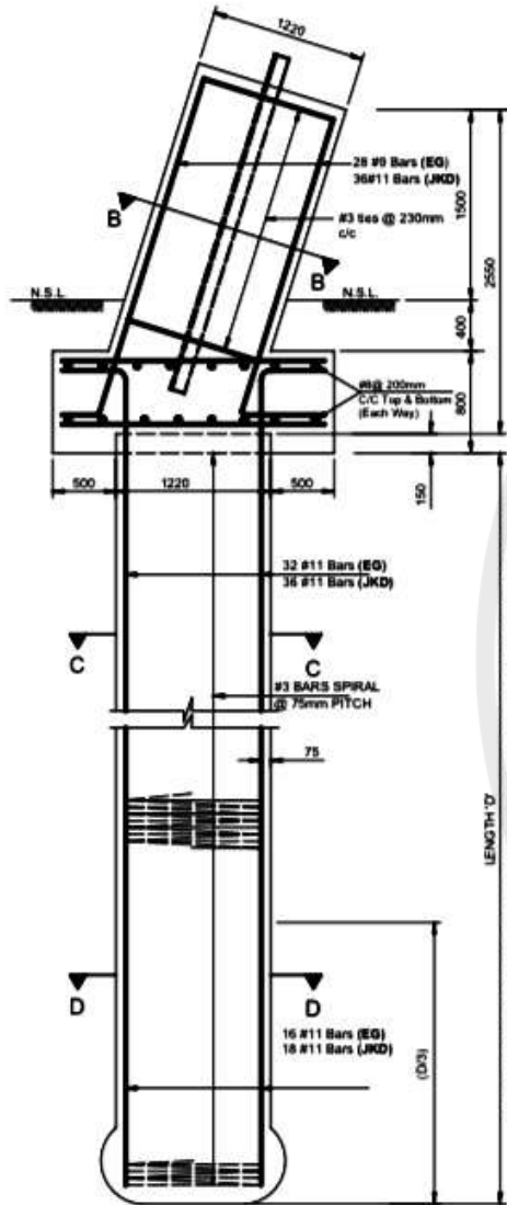
SECTION A-A
