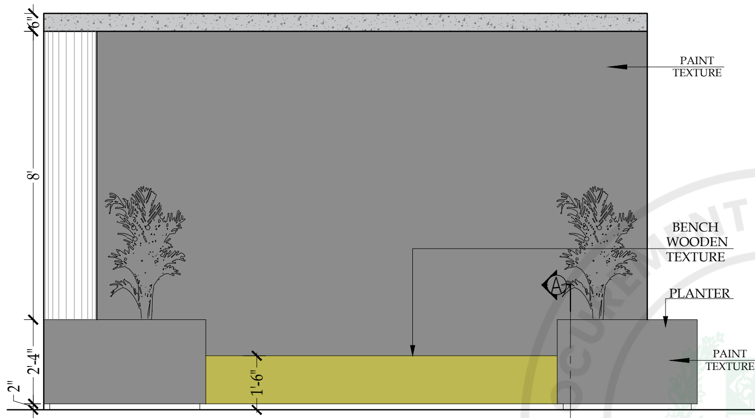
ELEVATION -3
