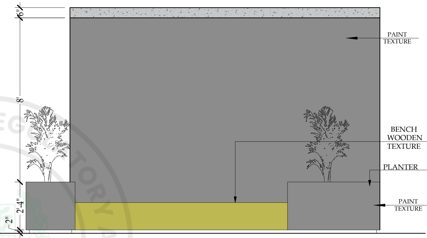
ELEVATION -4
