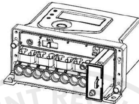
Step 2. Insert module to meter
